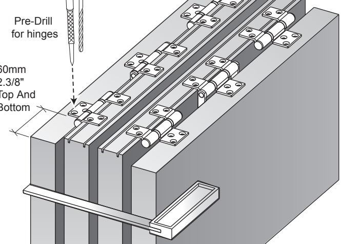
12. HINGES
