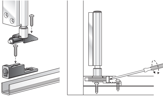
18. BOTTOM PIVOT BLOCK
