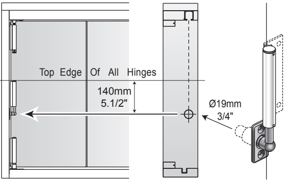
7. WALL PIVOTS
