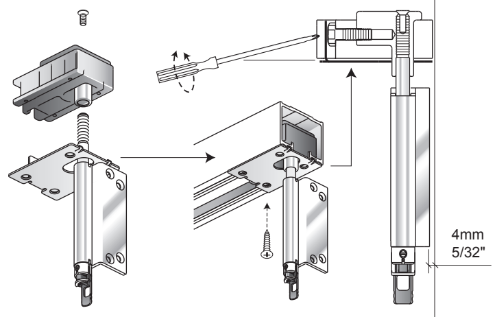
17. TOP PIVOT BLOCK
